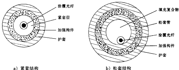
图 1 光缆结构示意图
